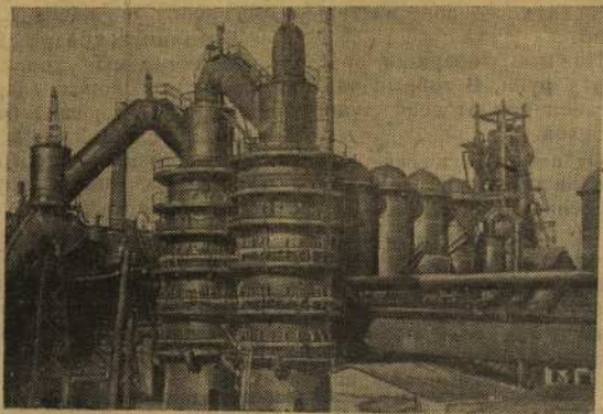
Восстановленная доменная печь № 3 Краматорского металлургического завода имени Куйбышева.
