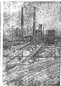
В ДНЕПРОДЗЕРЖИНСКЕ. Восстанавливаемый доменный пех Днепродзержинского металлургического завода имени Дзержинского.
